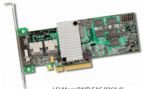
LSI MegaRAID SAS 9260-8i
