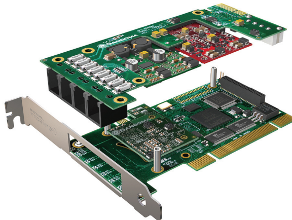
A200 FXO/FXS de cuatro puertos con el componente de cancelación de eco por hardware, desmontados.
